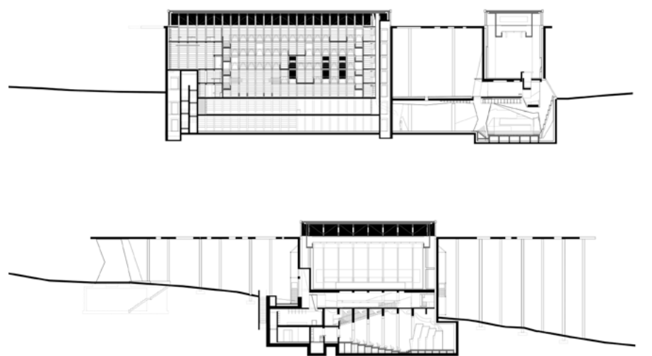
Querschnitte
