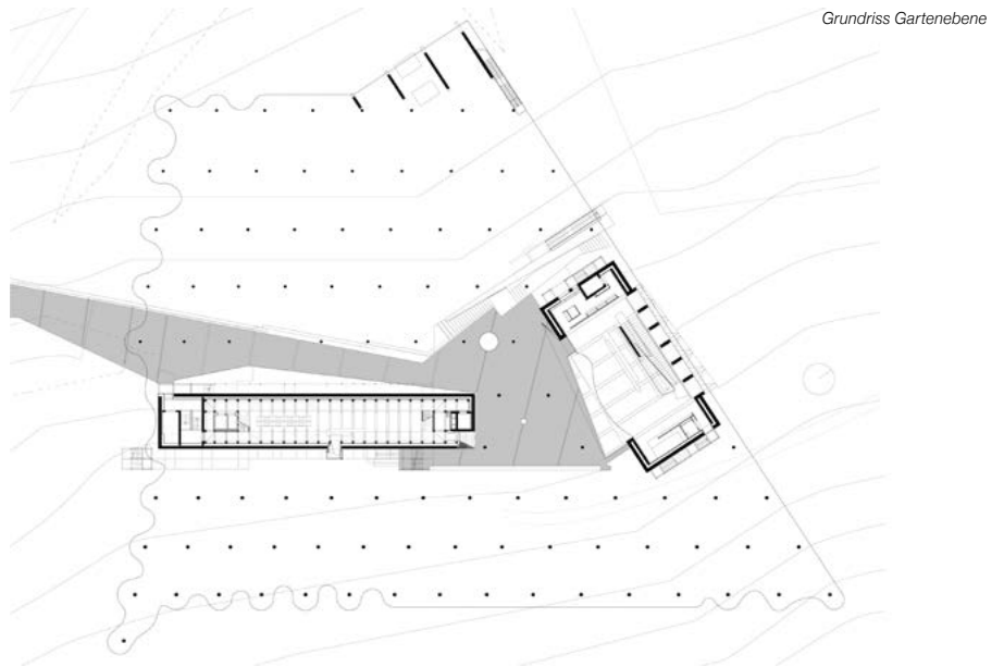
Grundriss Gartenebene
